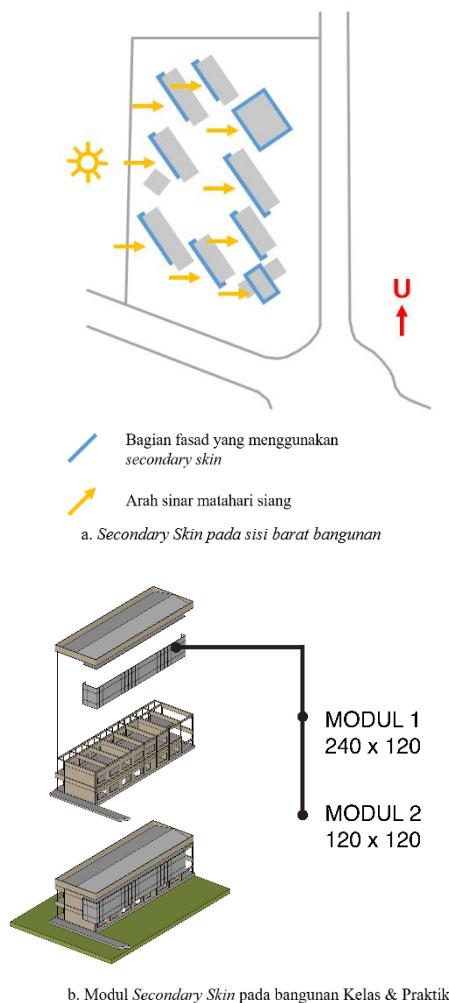
Gambar 14. Modul secondary skin dan penggunaan secondary skin
